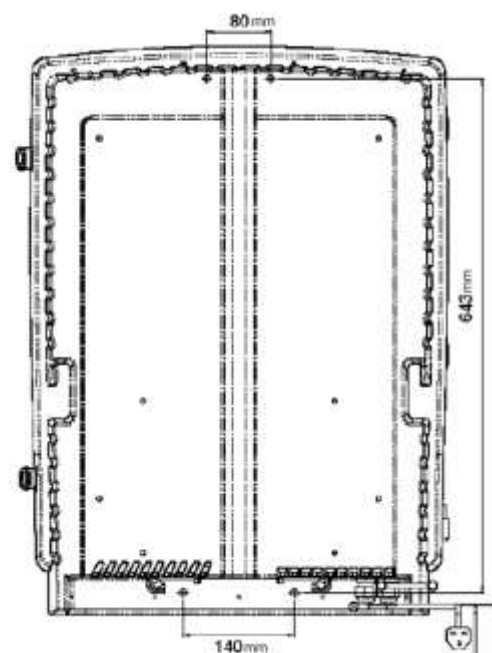
Hình 2 Kích thước mở
