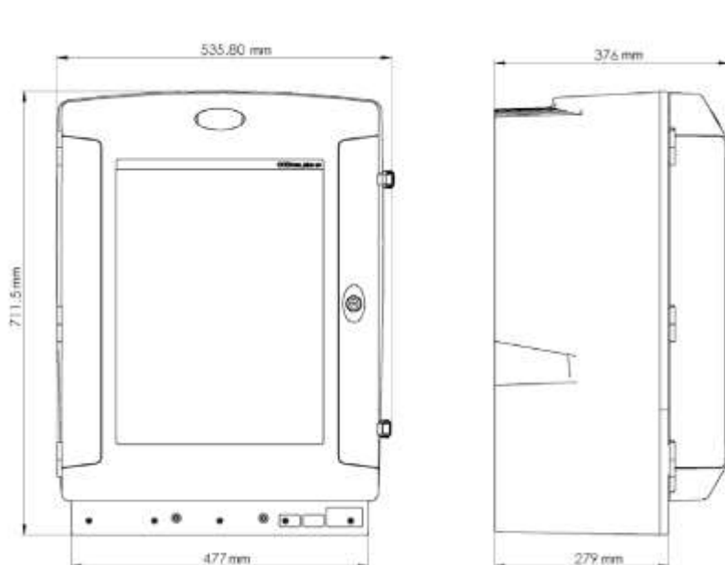
Hình 1 Kích thước vỏ thùng máy
